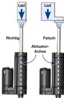
Abbildung 5 Exzentrische Last
