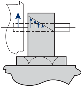
Abbildung 2 Freitragender Einbau
